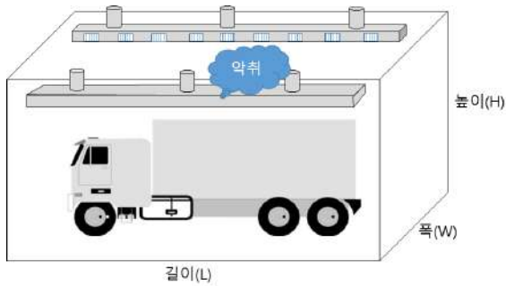
<그림> 출하시설 포집 덕트 설치방안
